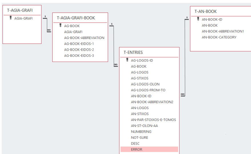
Εικόνα 1-Σχεσιακό Μοντέλο της Βάσης Δεδομένων
